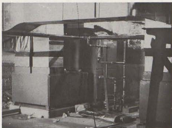
Aparelho de resfriamento e purificação do ar
